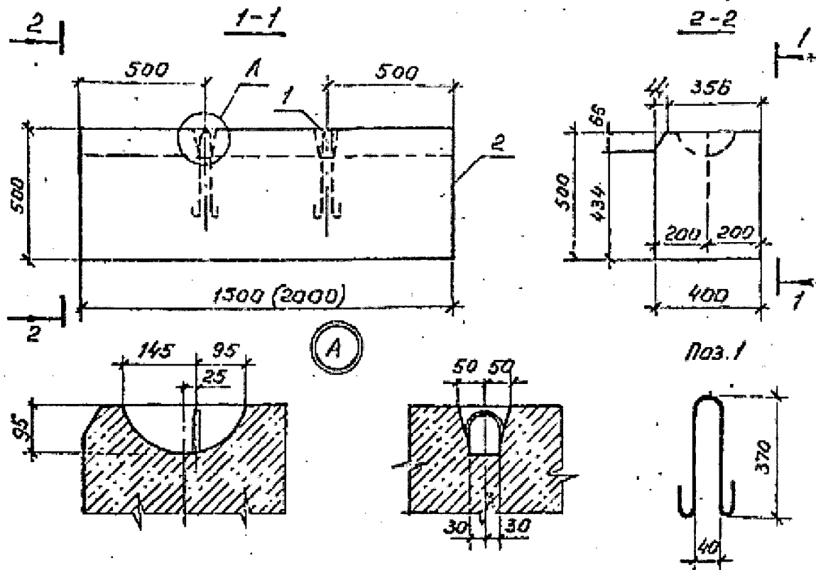
Рисунок 15 – Бетонный блок упора У-1
