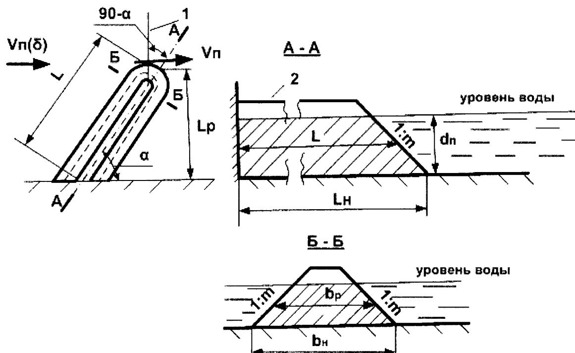
Рисунок 4 – Траверс у пойменной насыпи
