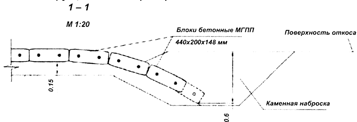
Рисунок А.2.4 – Возможные конструкции краевого участка защиты и заделки края крепления
