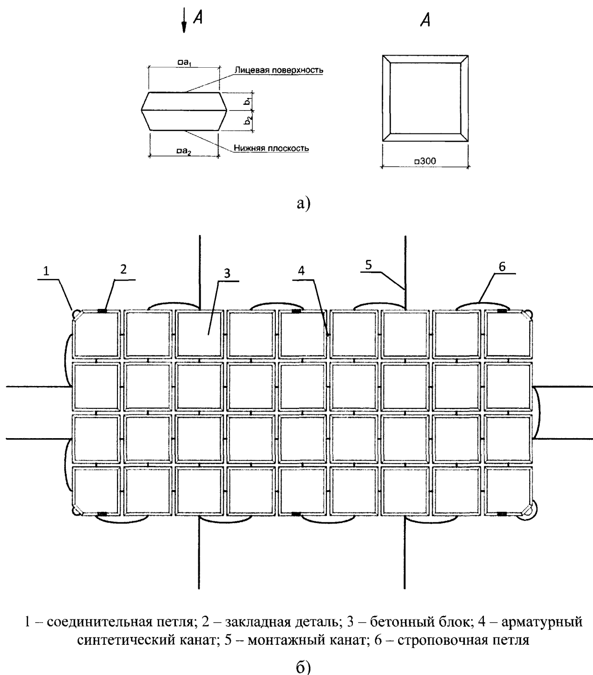
а) внешний вид бетонного блока КГПП; б) внешний вид плиты КГПП (вариант)
