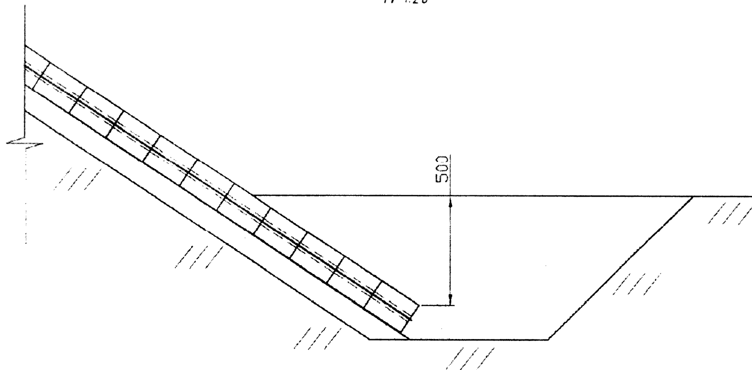
Рисунок А.2.5 – Возможная конструкция закрепления подошвы откоса
