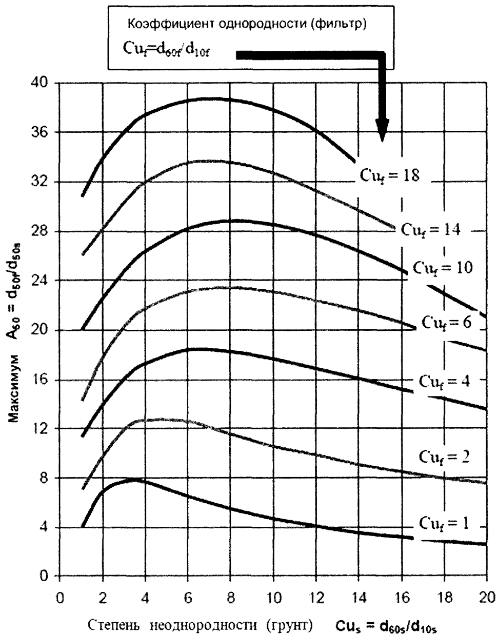
Рисунок 14 – График для подбора материала гранулированного фильтра
