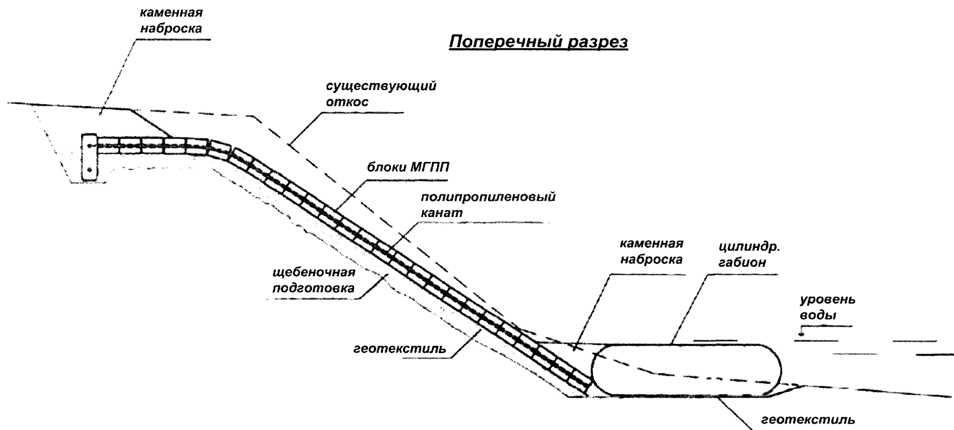
Рисунок А.2.6 – Вариант берегоукрепления. Поперечный разрез.
